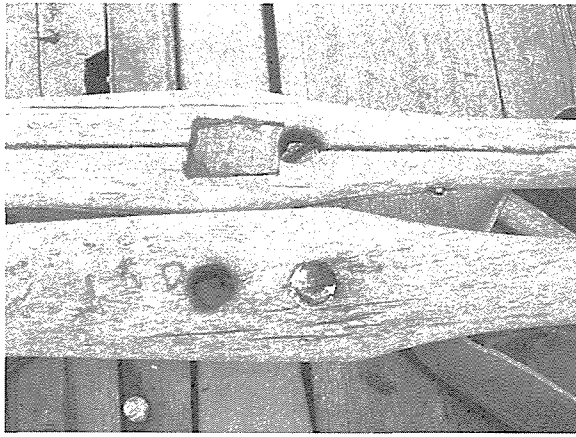
写真 47. 室蘭市イタンキ漁港 一材二穴車擧
