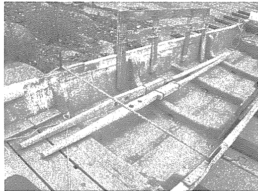
写真77. 2材（2穴）の車櫂 （2009年9月撮影稚内市宝来）
