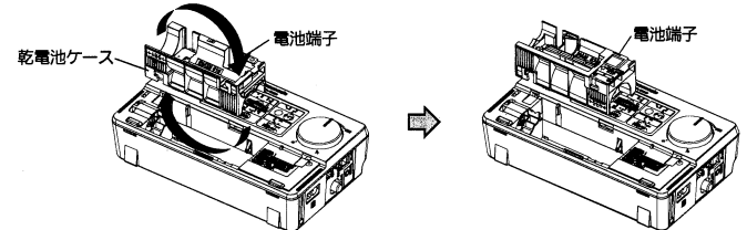
単1形乾電池
